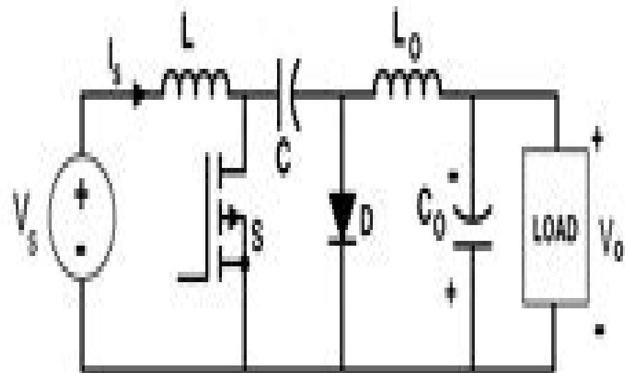
Cuk Converter
